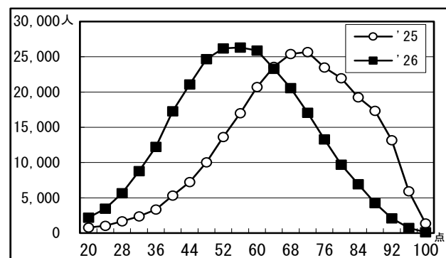
情報 I
