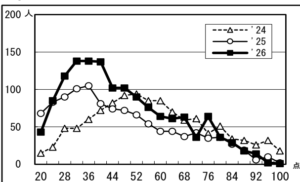
地学
