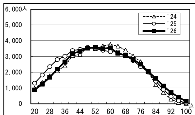
生物
