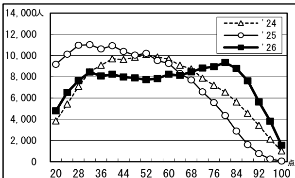
化学
