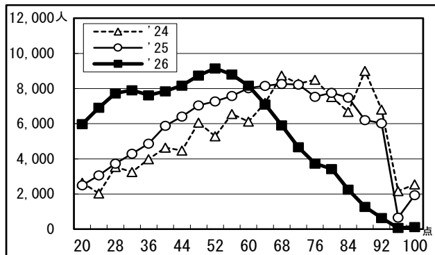
物理
